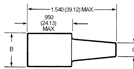
Receptacle P/N 120-1833-000
