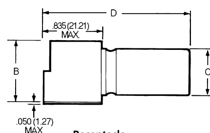
Receptacle
