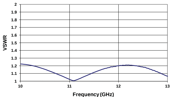
VSWR (10-13 GHz)
