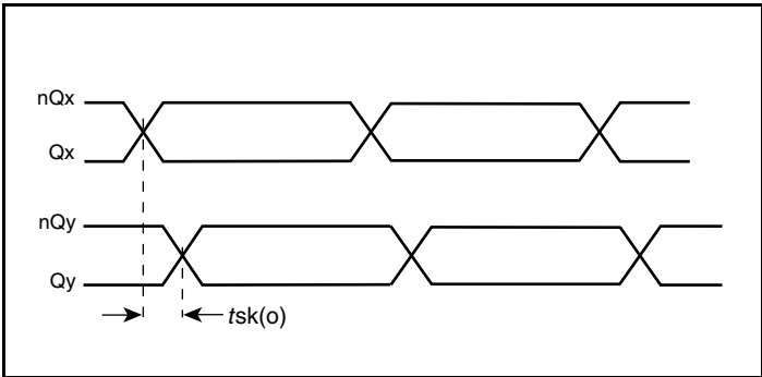
Output Skew
