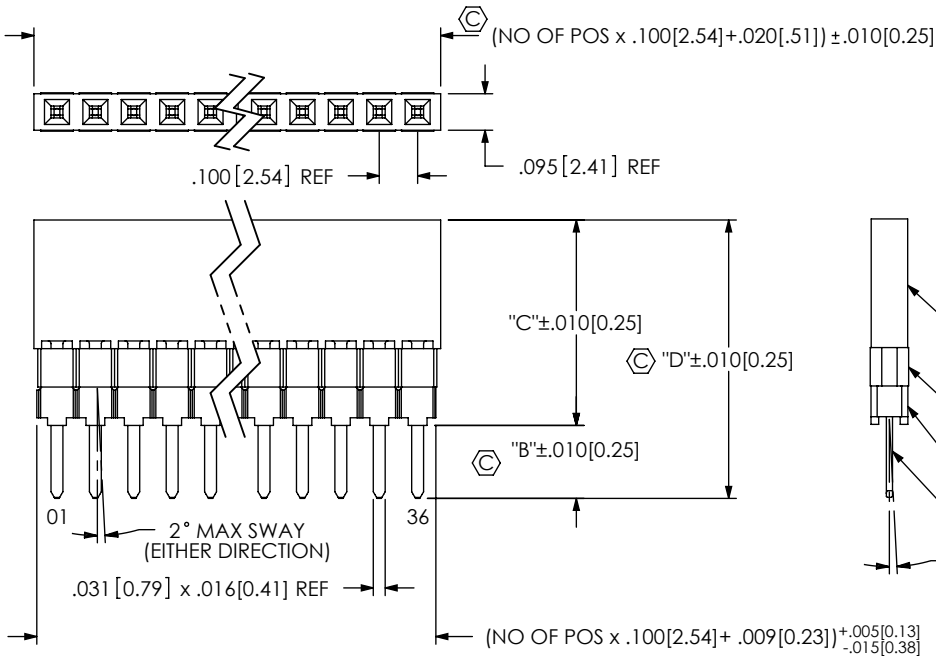
FIG 1 ESW-1XX-XX-X-S SHOWN
