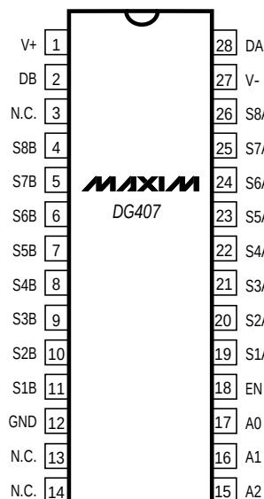
DIP/SO
