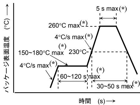
Pb フリーはんだ時の温度プロファイルー例
