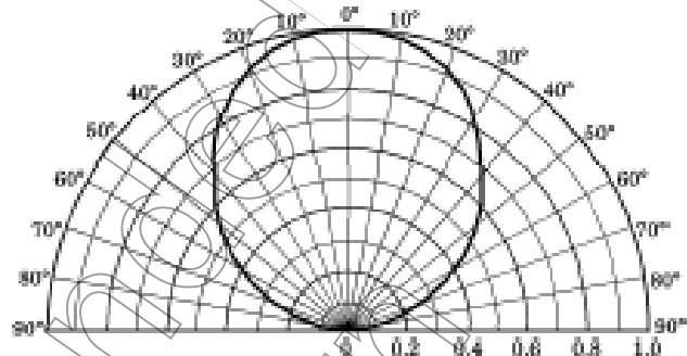
電極に対し垂直方向 T_a=25^\circ\text{C}
