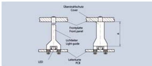
Einbaubeispiel · Mounting Example
