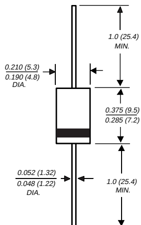
DO-201AD
