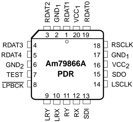
20-Pin PLCC
