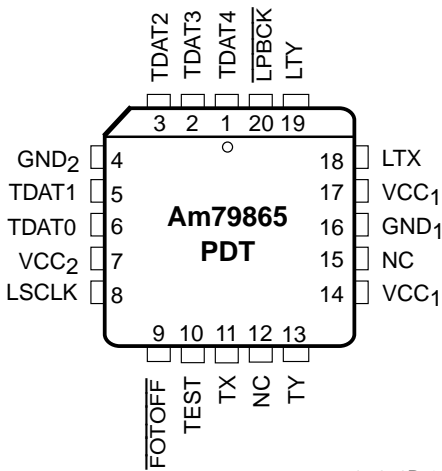
20-Pin PLCC
