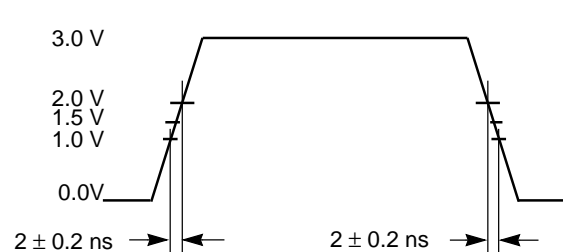
TTL Input Waveform
