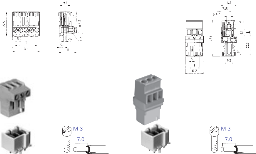
Type 8105 B/... C... OB
