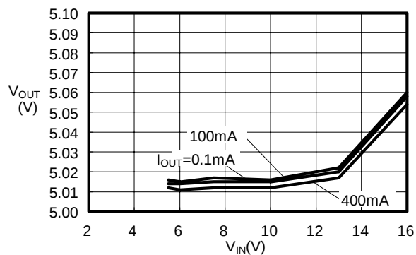
(12) V_{OUT}-V_{IN}
