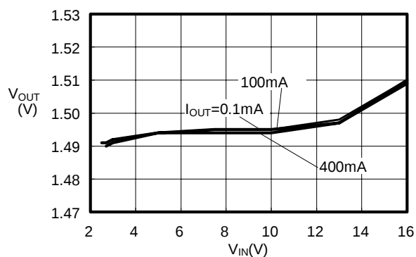
(10) V_{OUT}-V_{IN}
