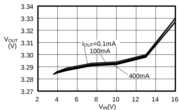
(11) V_{OUT}-V_{IN}
