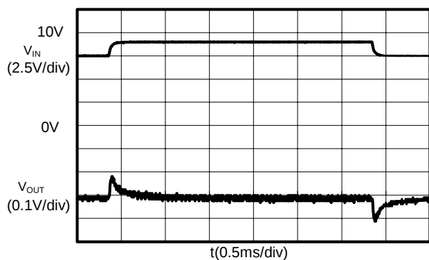
(5) S-8532B50AFT( I_{OUT} : 10mA)
