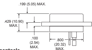
Receptacle
