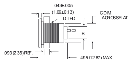
Receptacle
