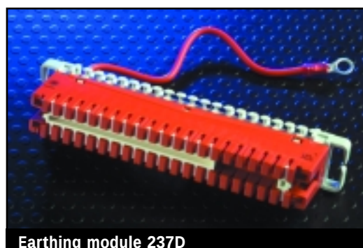
Earthing module 237D
