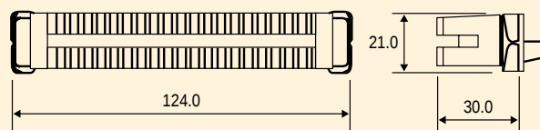
10 Pair Module
