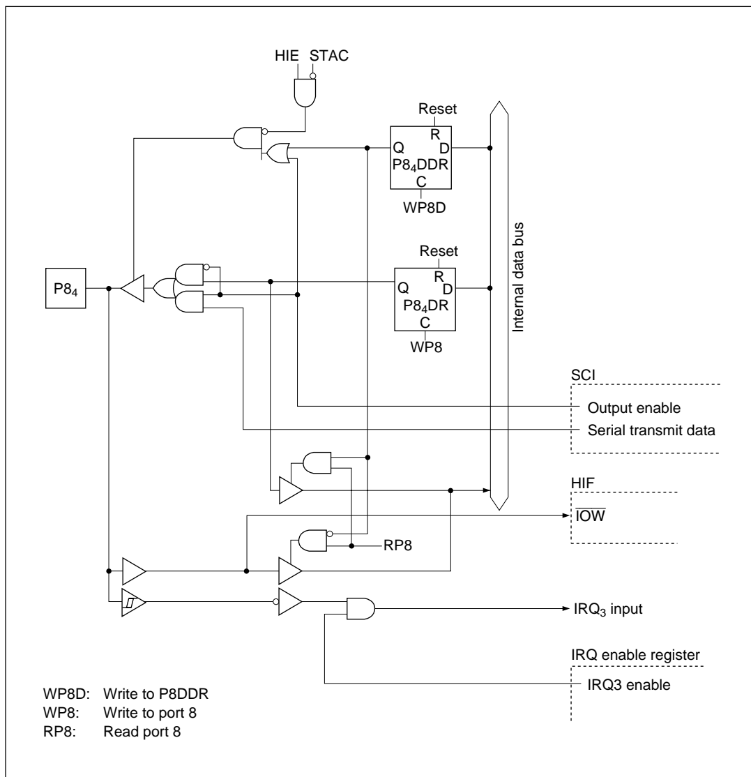
Figure C-8 (d) Port 8 Block Diagram (Pin P8 4 )
