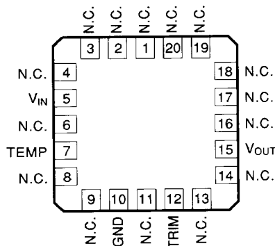
REF-01RC/883 LCC (RC-Suffix)
