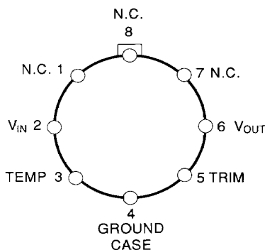
TO-99 (J-Suffix)
