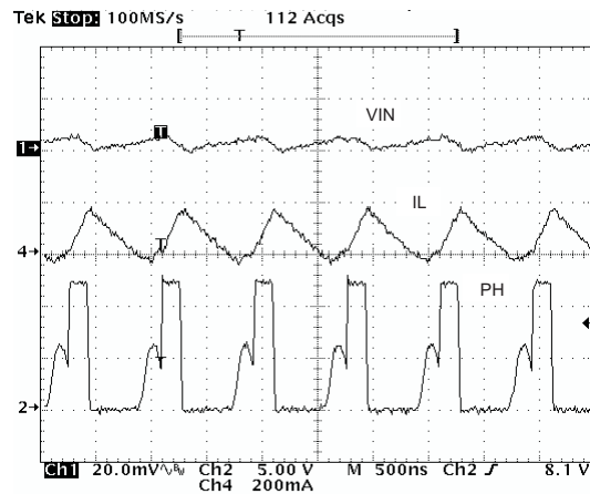
Figure 60. Input Ripple DCM
