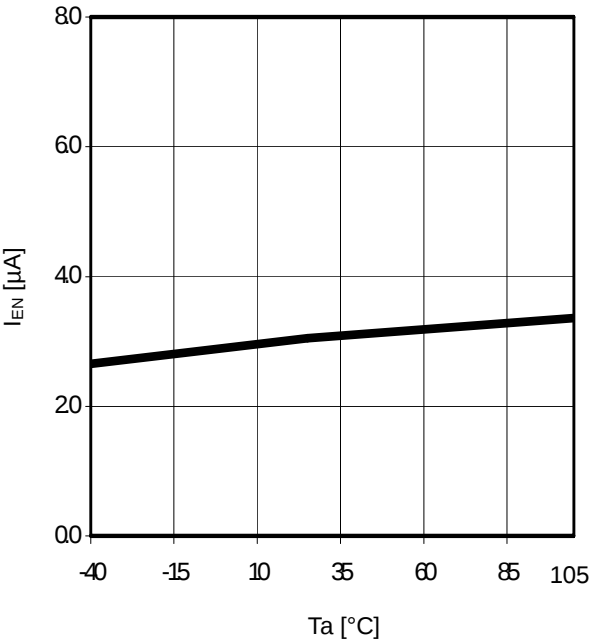
Fig. 24 Ta- I_{EN}
