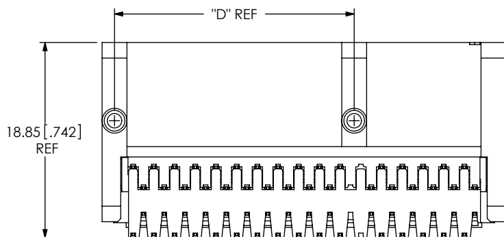
FIG. 1 (PCIE-064-02-X-D-RA SHOWN)
