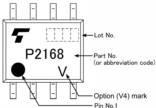
Fig. 16.3 Marking Example(Note)
