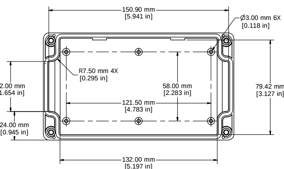
LID - INSIDE
