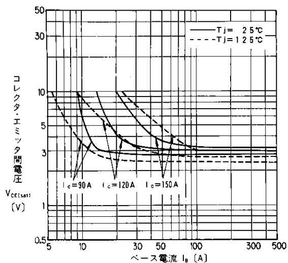
出力特性
