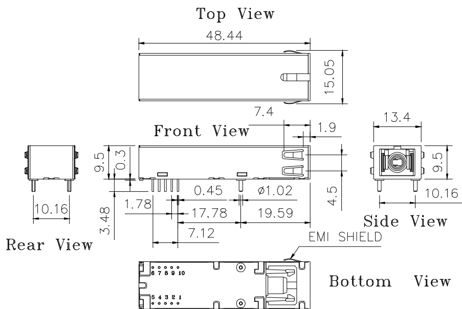
BTRS-5780E-1510G
