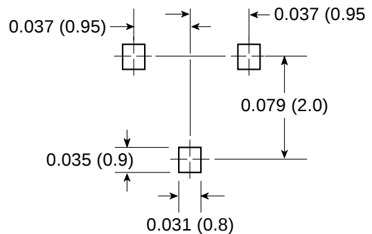
BAS40-06
