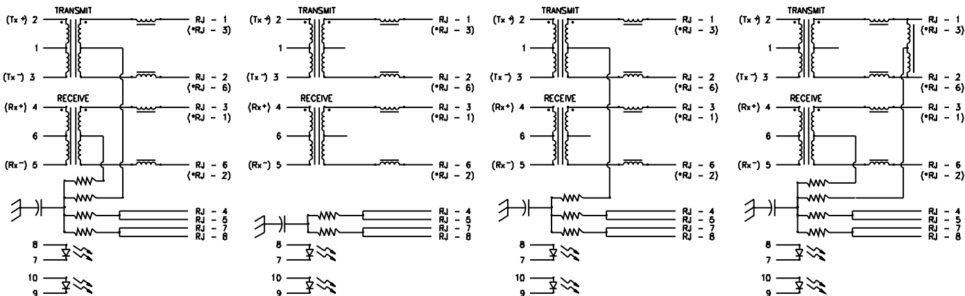
SCHEMATIC (RJMG-73xx-3x-01) SCHEMATIC (RJMG-73xx-8x-01)
