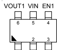
VOUT2 GND EN2 TSOT-23-6
