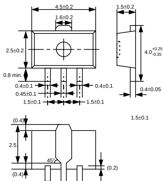
(2) SOT-89-3
