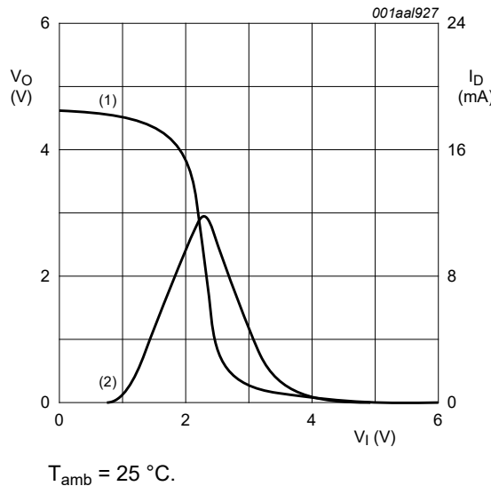
Fig. 9. V_{CC} = 4.5\text{ V} ; I_O = 0\text{ A}
