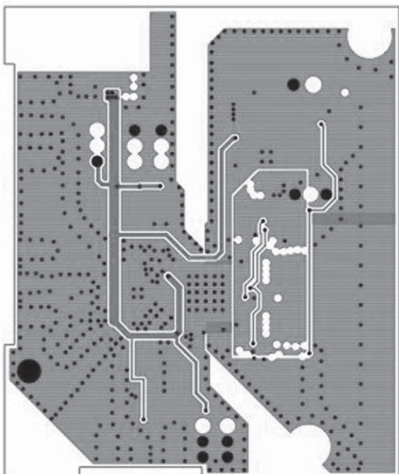
Inner Layer 3
