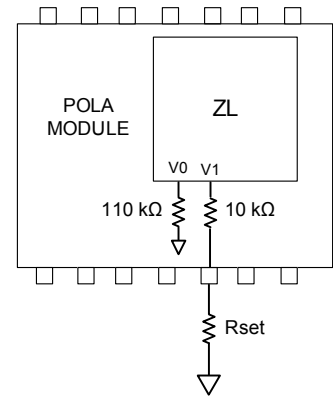
FIGURE 11. R_{SET} on a POLA Module
