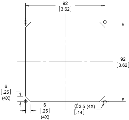
CUTOUT DIMENSIONS
