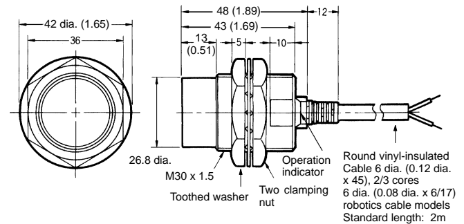
Fig. 8: E2E-X18MY□-N
