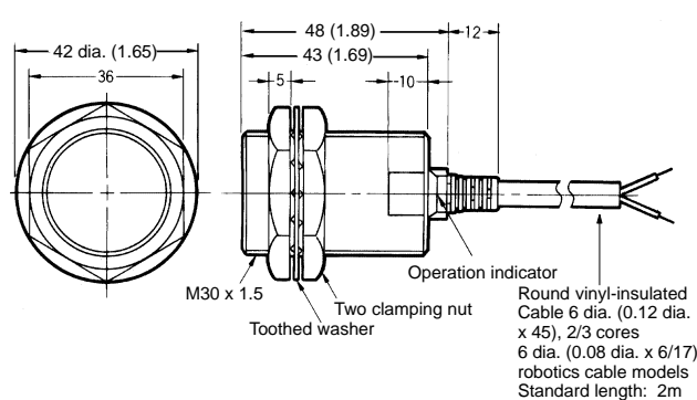
Fig. 7: E2E-X10Y□-N
