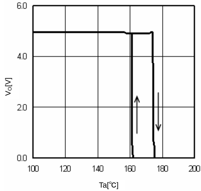
Fig.16 TSD ( I_O=0\text{mA} )
