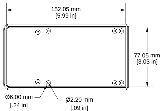
LID - INSIDE
