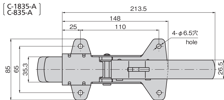
C-835-B (埋込タイプ) Embedded type
