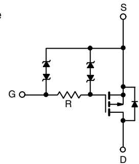
P-Channel MOSFET
