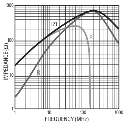
MZ 1608- 601Y
