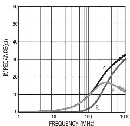
MU 1005- 121Y
