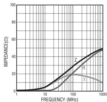
MU 1005- 151Y
