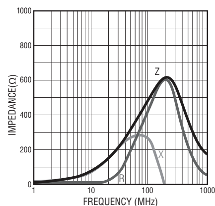
MG 1608- 152Y
