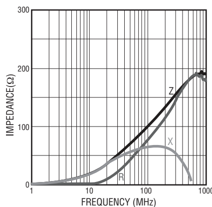
MU 1608- 221Y
