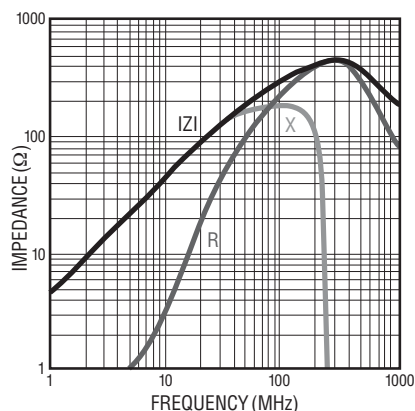
MZ 1608- 102Y
