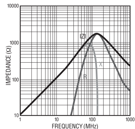
MG 1608- 152Y
