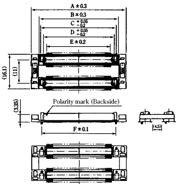
Unit:mm
