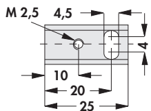
SK 12 SA 32 30 K/W 1 x SOT 32
