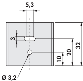
UK 35 SA 32 SOT 32
