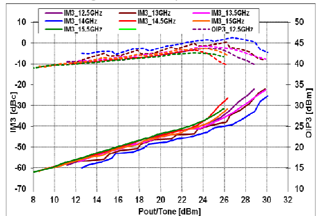
@Vds=6V, Ids=2500mA
