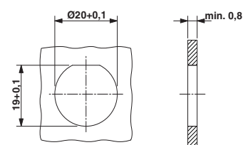
RC-00000006100, Montage Bohrung mit Verdrehenschutz und Kontermutter (Empfehlung bei Einbau in Stahlblechwand)
