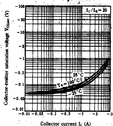
V_{CE(sat)} - I_C
