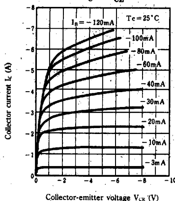
I_C - V_{CE}
