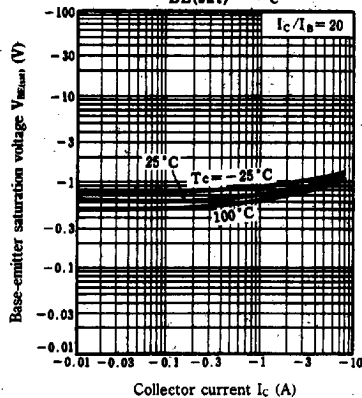
V_{BE(sat)} - I_C
