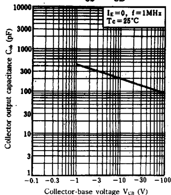
C_{ob} - V_{CB}
