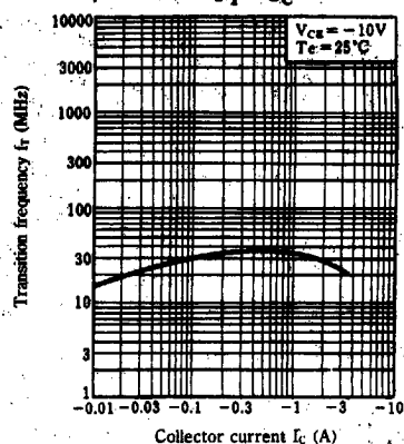
f_T - I_C
