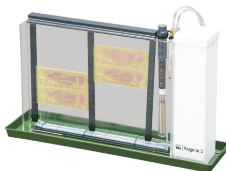
Ätzgerät 2
