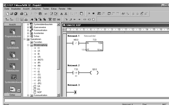
Bild 2-8 Netzwerk 2
