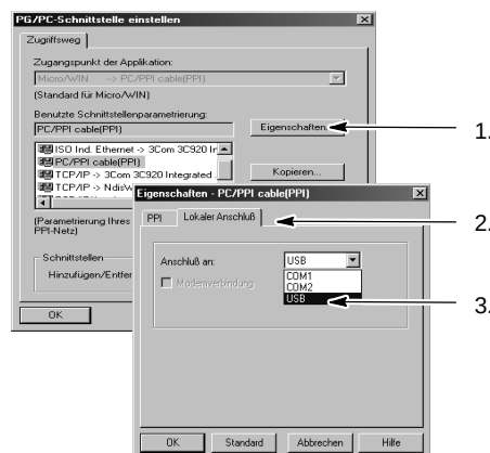
Bild 7-2 Auswahl des PPI-Multi-Master-Kabels
