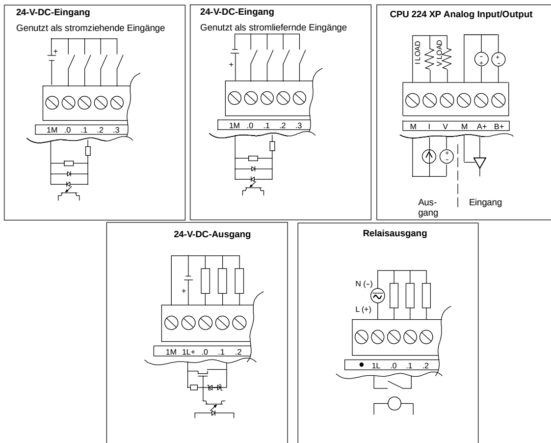
Bild A-2 Eingänge und Ausgänge der CPU
