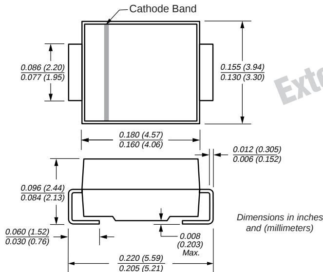
DO-214AA (SMBJ-Bend)
