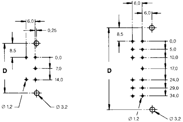
180°-Ausführung/Vertical
