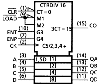
TC74HC161A
