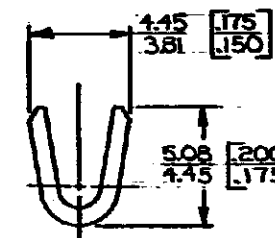
SECT A-A
