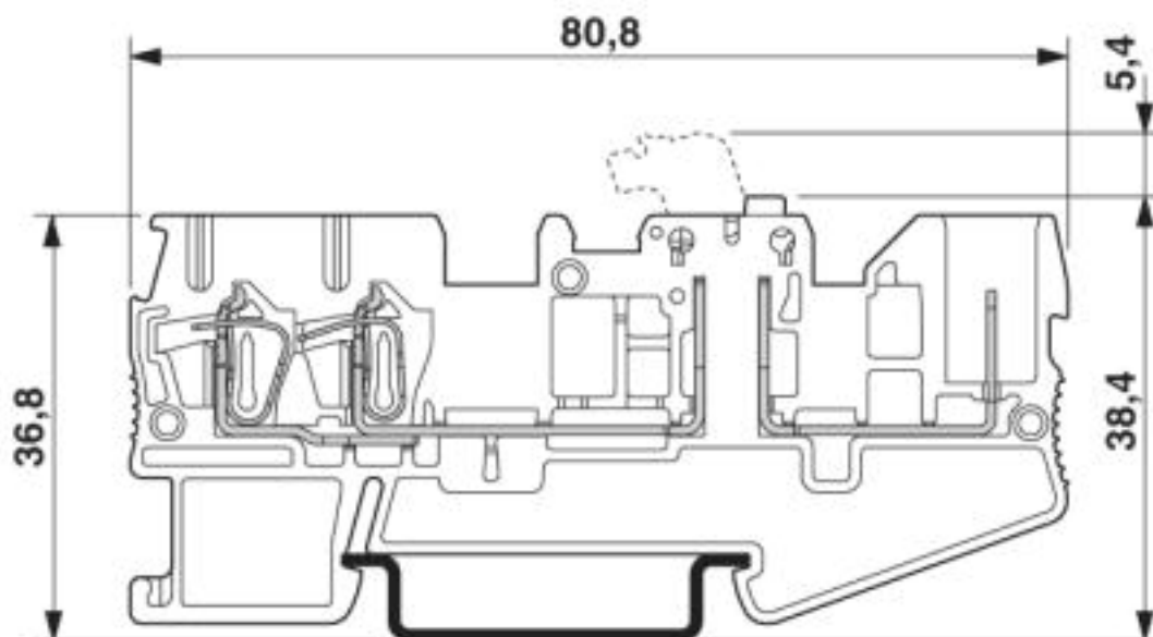
Maßzeichnung
