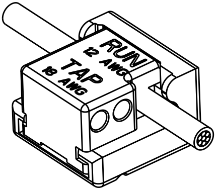
SCALE 2:1
