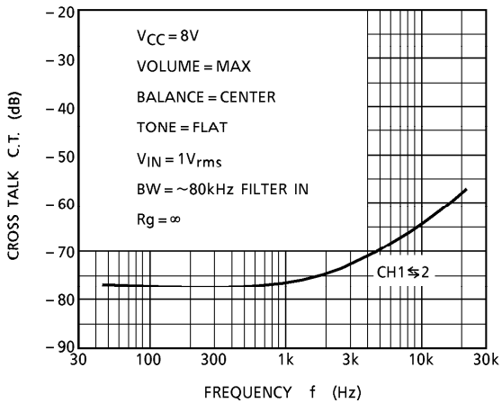
C.T. - f
